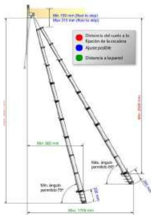
Medidas Loft 270
